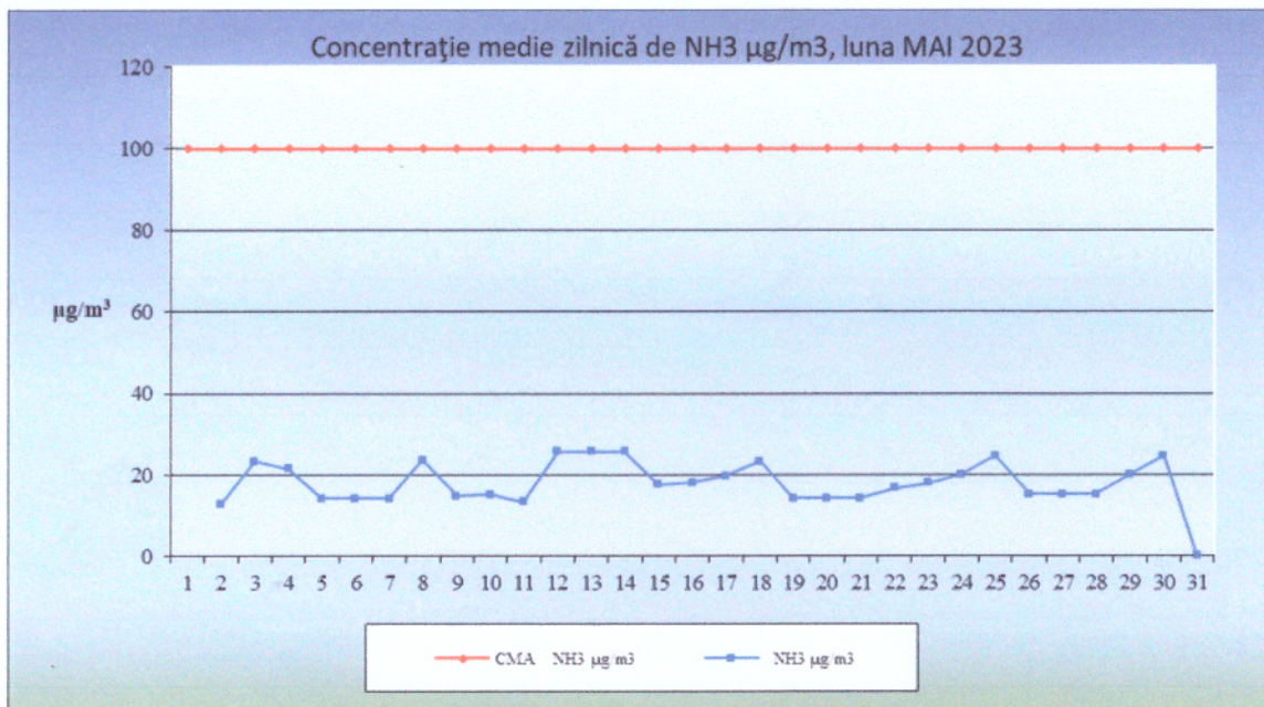
Figura 3. Evoluția concentrației medii zilnice de \text{NH}_3
