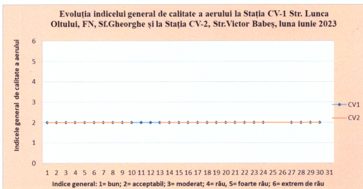
Figura 2. Evoluția indicelui general de calitate a aerului
