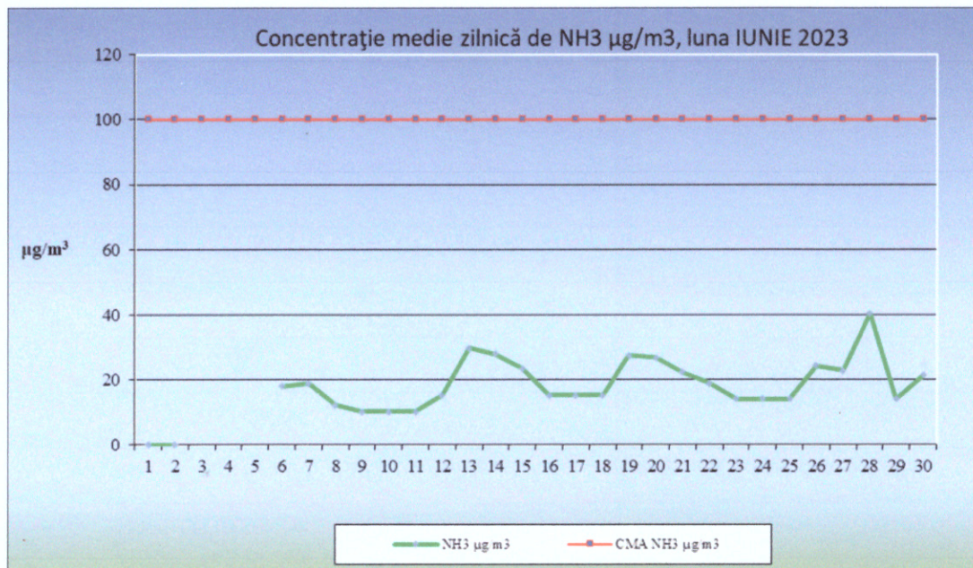
Figura 3. Evoluția concentrației medii zilnice de \text{NH}_3
