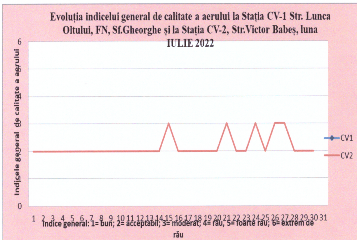
Figura 2. Evoluția indicelui general de calitate a aerului
