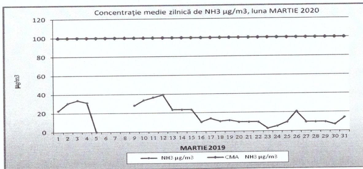
Figura 2. Evoluția concentrației medii zilnice de NH 3
